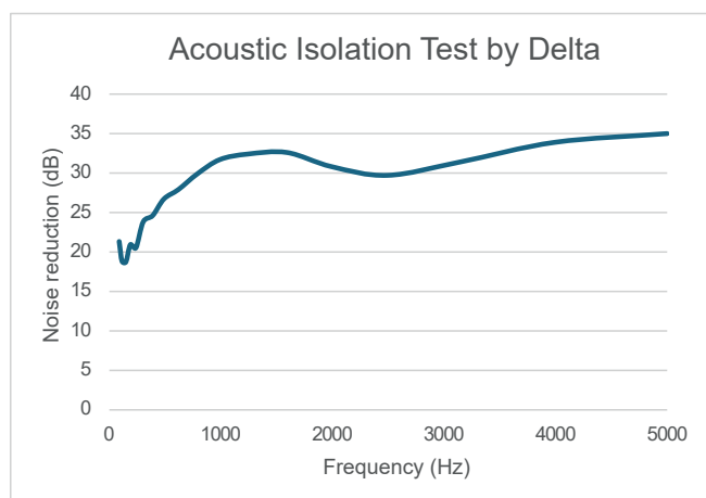
Typisk dæmpningseffekt af Miljøskærms støjskærms element
